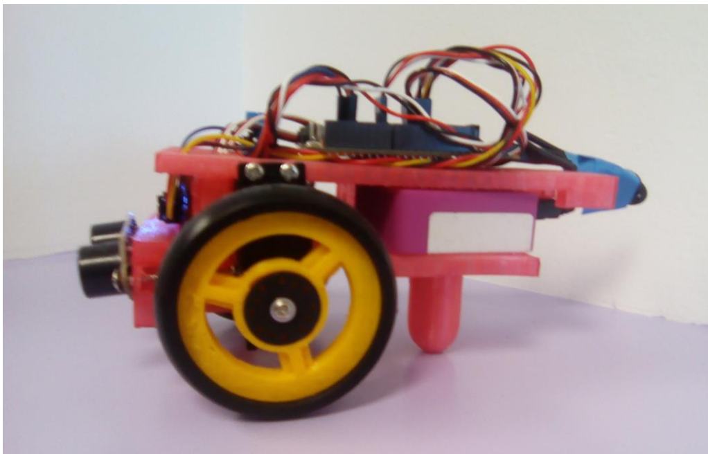
Original vehículo que se dirige desde un móvil y evita obstáculos. Estructura diseñada por un alumno de 2º de ESO.
